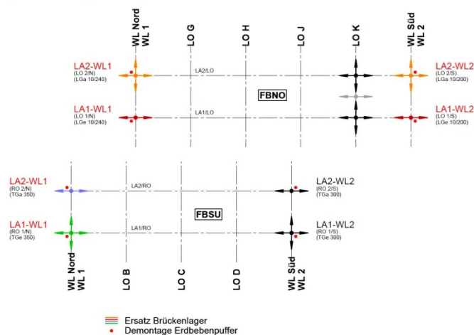
Schema Lagerersatz
